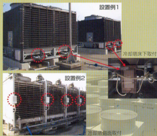
冷却塔側面取付
